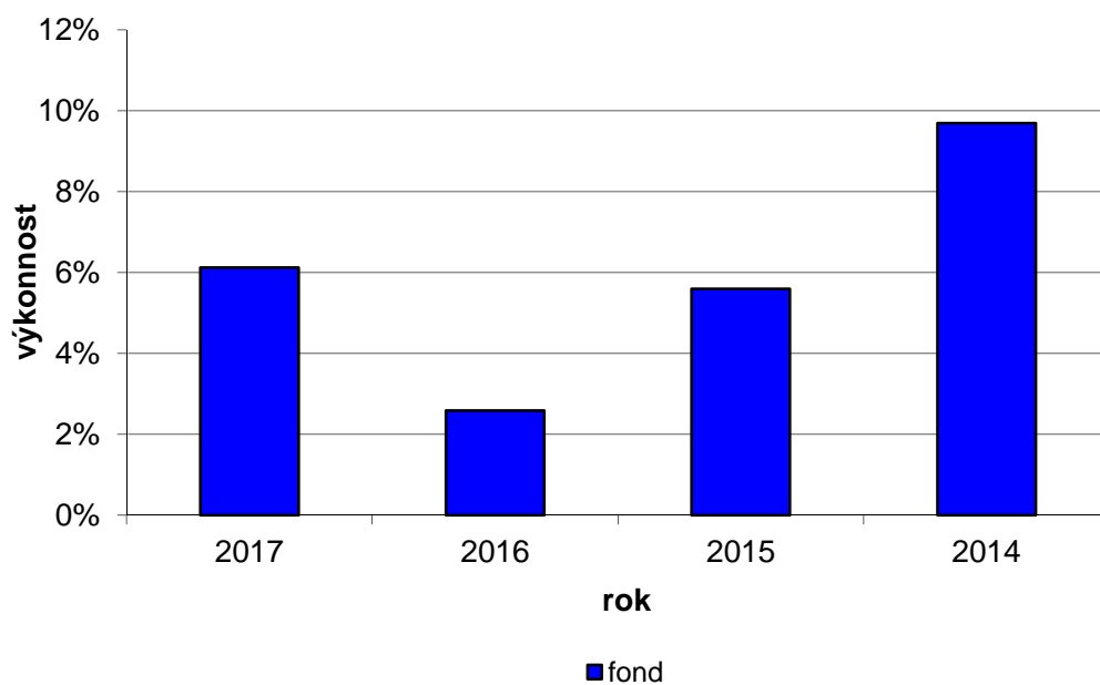
Výkonnost Amundi CR All-Star Selection (I)
