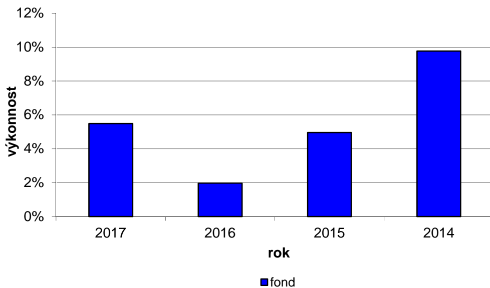
Výkonnost Amundi CR All-Star Selection (I)
